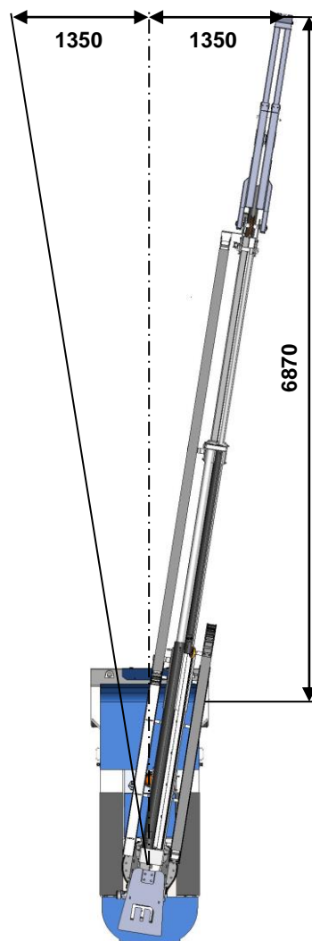
Option couronne d'orientation 18° (2x9°)
